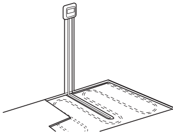
Рисунок 5. Пример расположения терморегулятора и датчика температуры.
